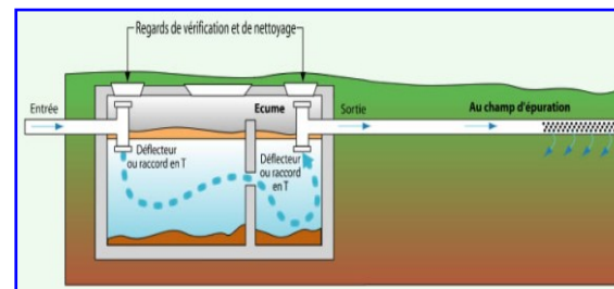
Fosse septique
